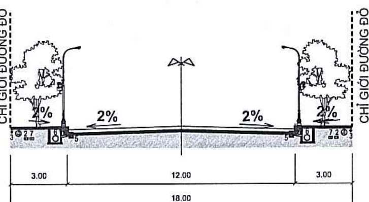
MẶT CẮT C-C
