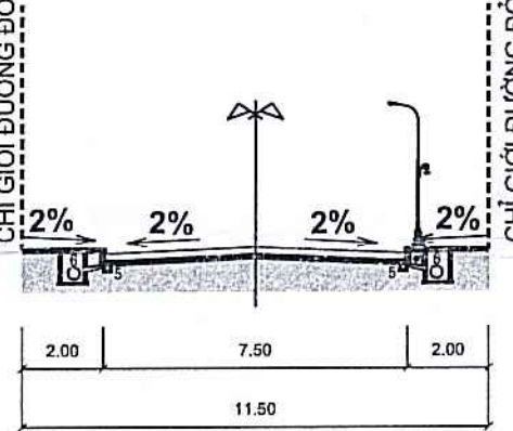
MẶT CẮT 5-5
