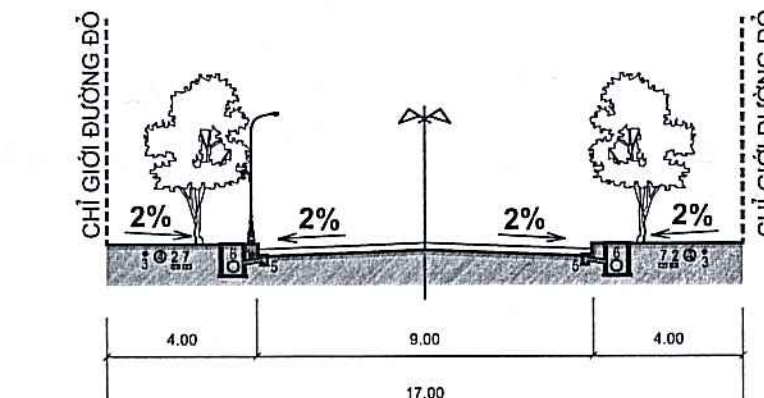
MẶT CẮT 2-2
