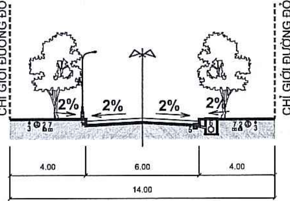
MẶT CẮT 4-4
