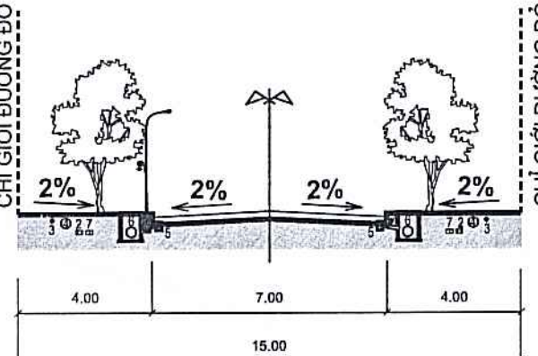
MẶT CẮT 3-3
