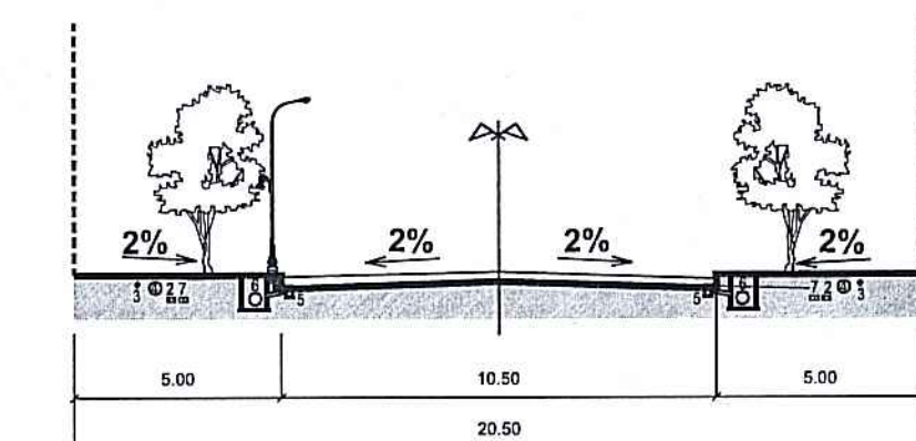
MẶT CẮT 1-1
