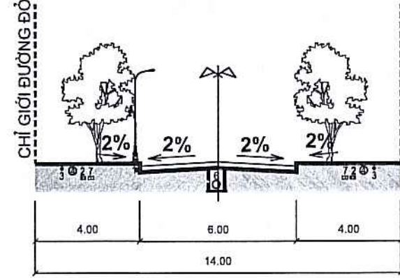
MẶT CẮT 4-4 (ĐOẠN CỎ CỐNG HỘP 2X1.5M)
