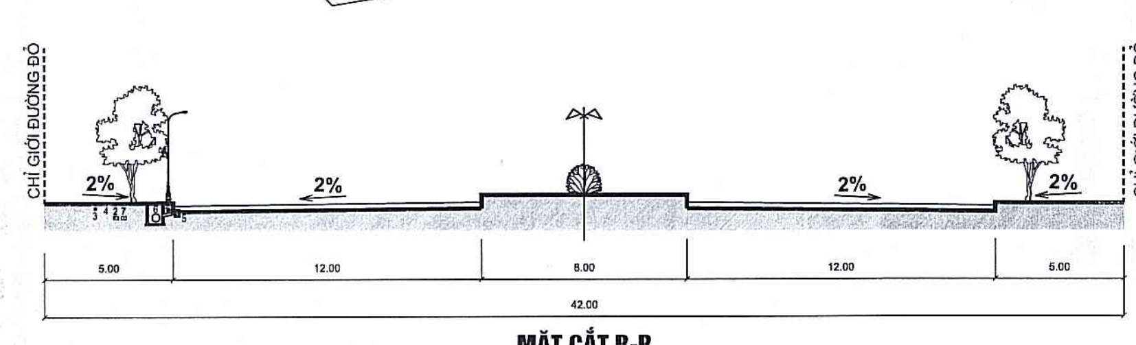
MẶT CẮT B-B
